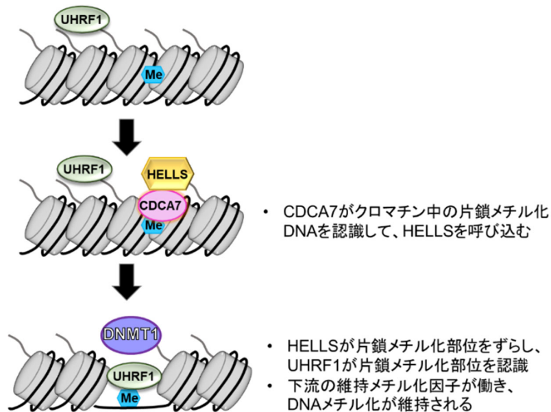
図 2：本研究で明らかにしたヘテロクロマチン領域の DNA 維持メチル化の新しい分子機構
