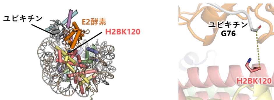
図 2 ユビキチン化反応が起こる状態の仮想モデル (反応に必要な E2 タンパク質をオレンジ色で、ユビキチンを灰色で示す)。左：全体構造。右：H2BK120 のクローズアップ図。ユビキチン化において共有結合が形成されるユビキチンの 76 番目のグリシンが H2BK120 の近くに存在する。
