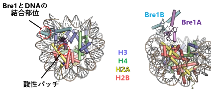
図 1 Bre1 複合体がヌクレオソームに結合した構造 (2 方向で示す)
