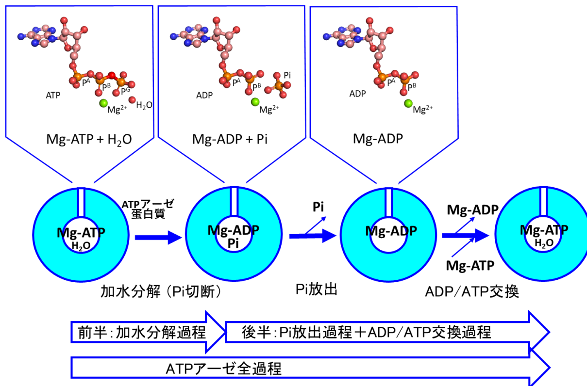
図 3. ATP アーゼ蛋白質は ATP アーゼ過程によって蛋白質分子内に結合した ATP を加水分解し(前半過程)、さらに分解産物(Pi と ADP)を放出する(後半過程)。上段は、Mg-ATP, Mg-ADP-Pi, Mg-ADP の構造:炭素(桃色)、窒素(青)、リン(朱)、酸素(赤)の各原子と \text{Mg}^{2+} (緑)。
