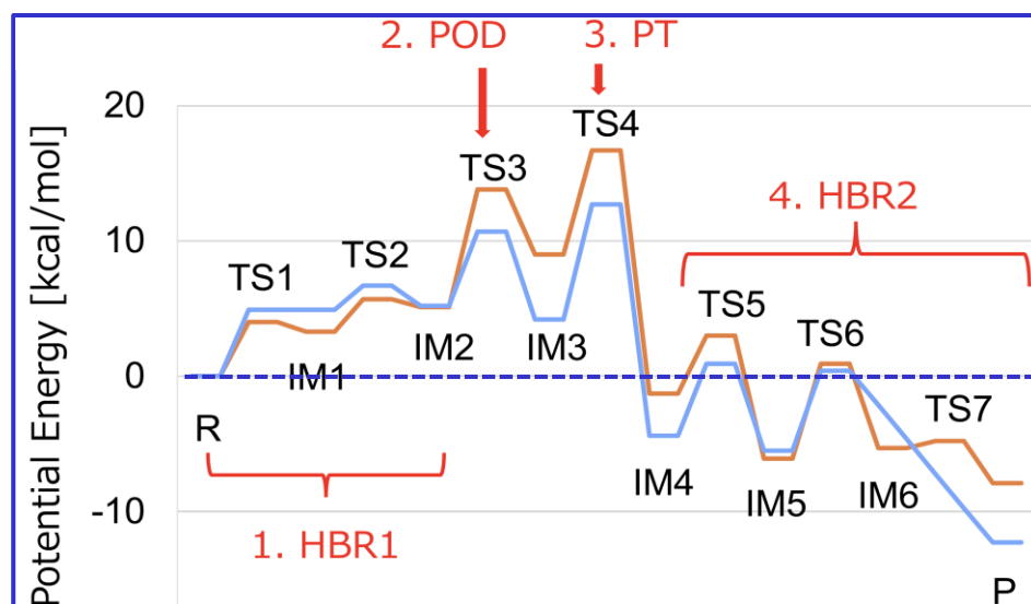
図 2. F 型アクチンの ATP 加水分解反応の反応経路に沿ったポテンシャル・エネルギー・プロファイル。反応の始状態 (R:ATP 結合状態)、反応中間状態 (IM)、遷移状態 (TS)、と反応の終状態 (P:ADP-Pi 結合状態)。始状態の構造から出発して終状態に至る計算結果はオレンジで、終状態の構造から出発して始状態に至る計算結果は青で示す。2 つのエネルギー・プロファイルが大きく解離しないこと、さらに計算で得られた始状態・終状態の構造が、それぞれ実験で得られた構造とよく近似していたことは、解明された反応経路がよく辻褄があっていることを示す。反応過程全体は 4 ステップ(赤表示)に区分できる。
