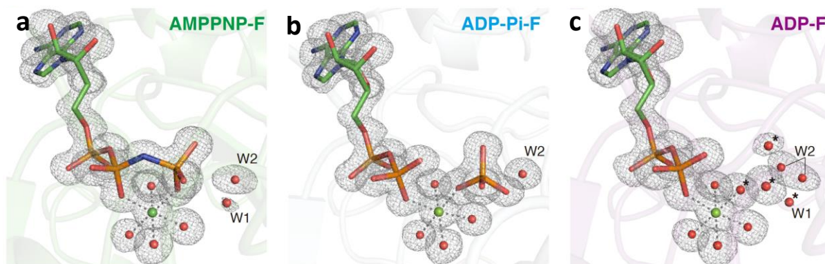
図 1.F 型アクチンの高分解能結晶構造(1.15 Å 分解能)の部分。いずれもアクチン蛋白質内に結合した (a) AMPPNP(ATP の構造アナログ)(b) ADP-Pi (c) ADP 各分子とその周辺の \text{Mg}^{2+} (緑色の球)、水分子の酸素原子(赤色の球)を示す。カゴ状の表示は電子密度分布、点線は \text{Mg}^{2+} の回りの配位結合。棒と球は、電子密度分布を基に置いた構造モデル。
