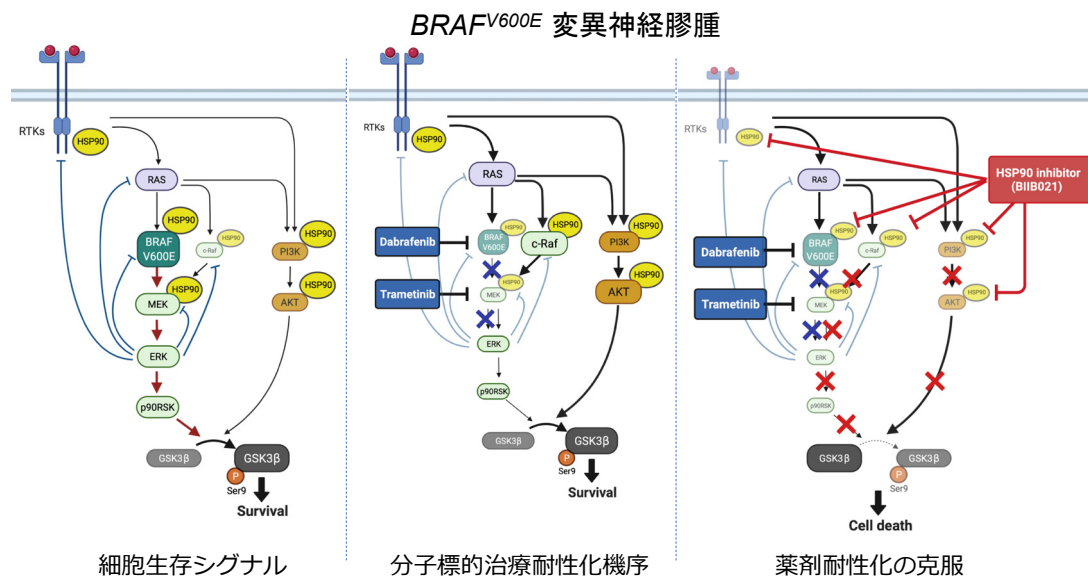
図 4 分子標的治療耐性化機序と耐性化克服のための治療アプローチ
