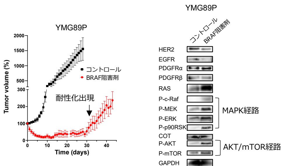
図2 BRAF^{V600E} 変異神経膠腫動物モデルを用いた腫瘍制御効果(左)と治療によるタンパク質発現変動 (右)
