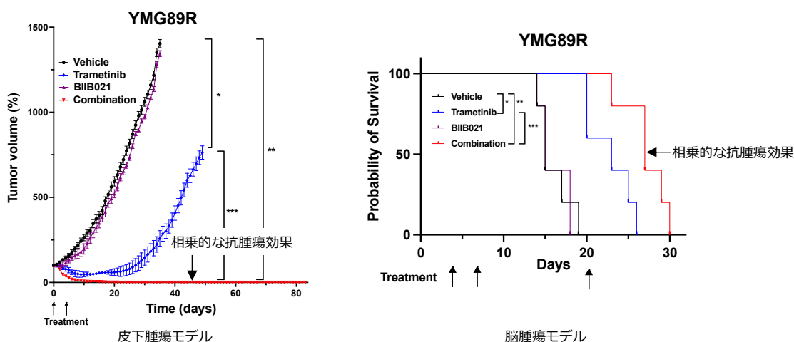
図 3 動物モデルを用いた MEK 阻害剤と HSP90 阻害剤併用による抗腫瘍効果の検証
