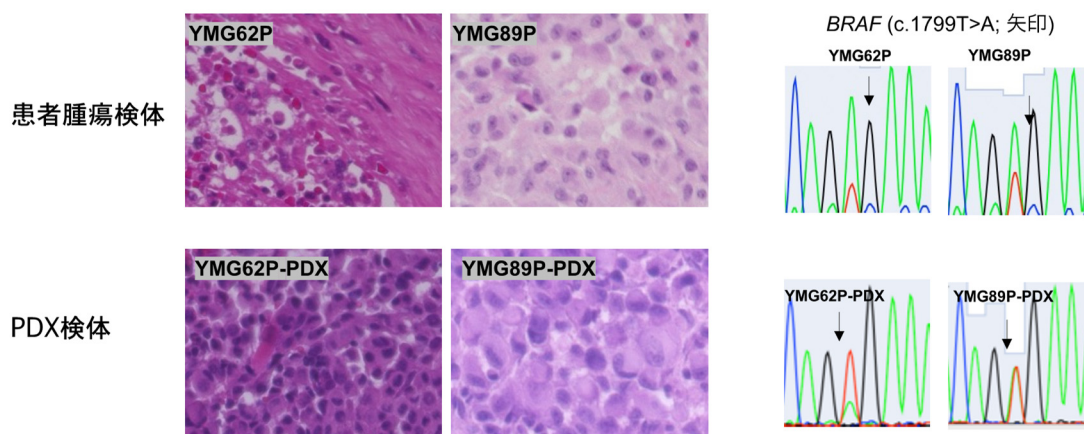
図1 BRAF^{V600E} 変異神経膠腫検体と再現性の高いPDXモデル（ヘマトキシリンエオジン染色と BRAF^{V600E} 変異解析）
