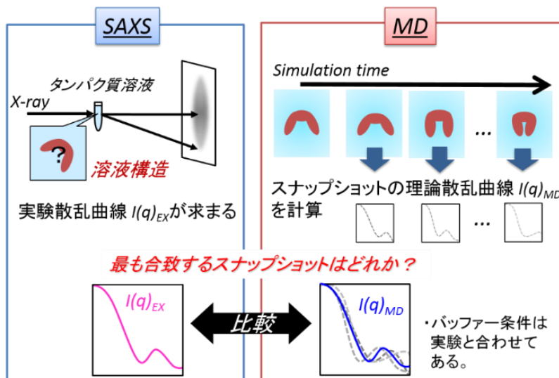
(図 2) SAXS-MD 解析の概要
