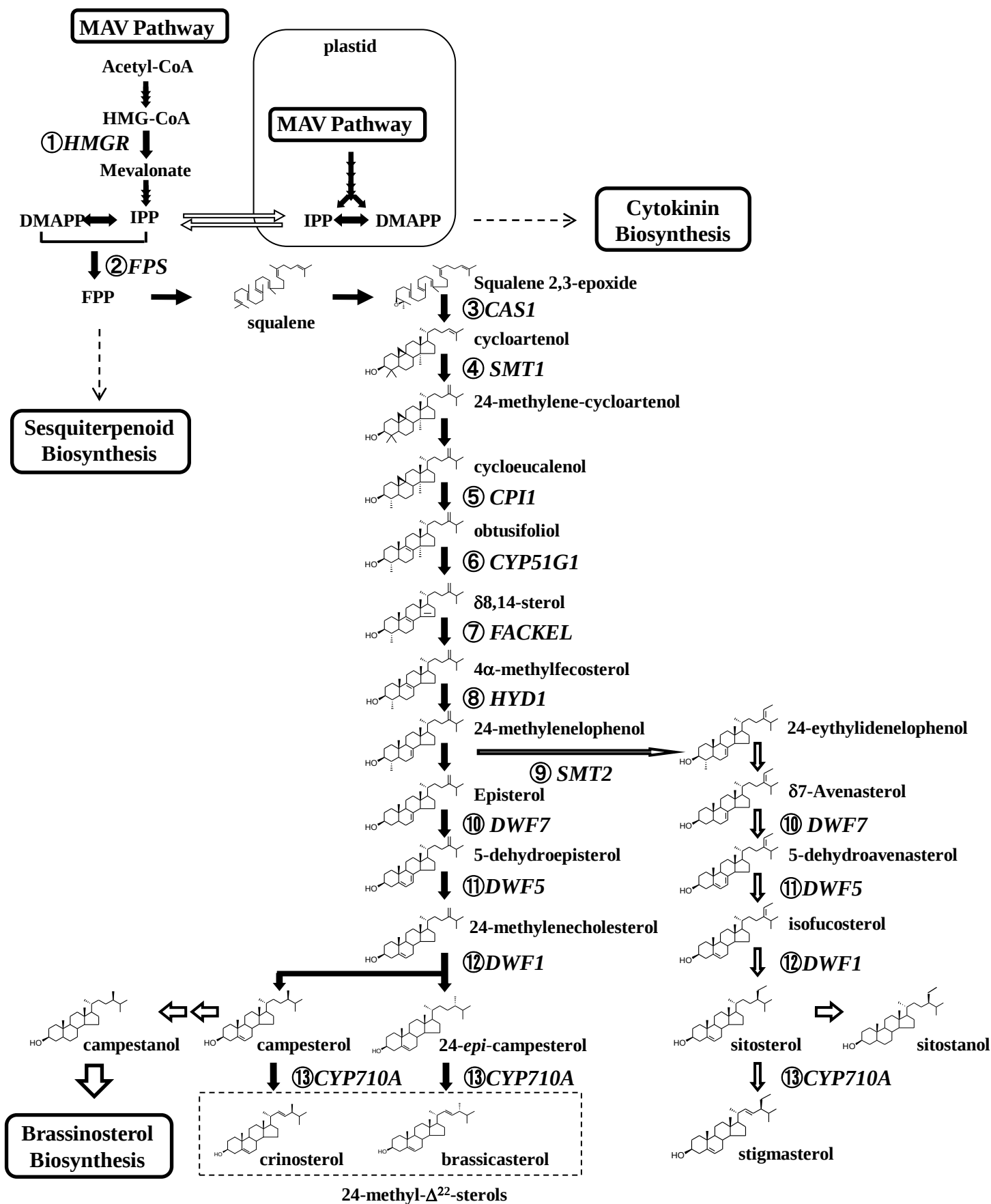
図1. 植物ステロール生合成経路
