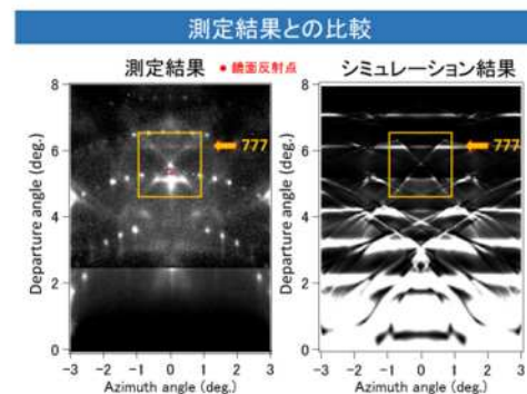
図1 Si(111)表面の菊池像の実測とシミュレーション結果
