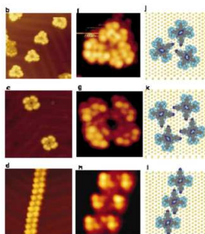
Si(111)
