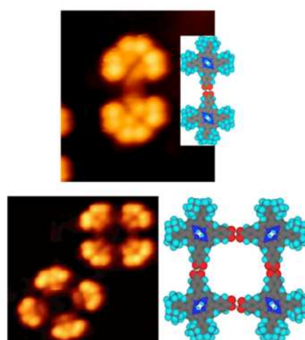
Au(111)
