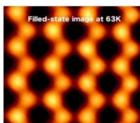
Si(001)
