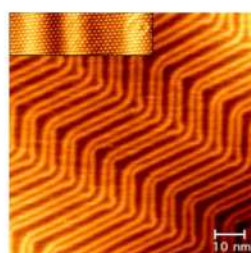
Au(111)
