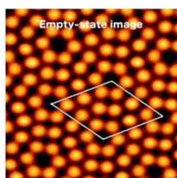
Si(111)
