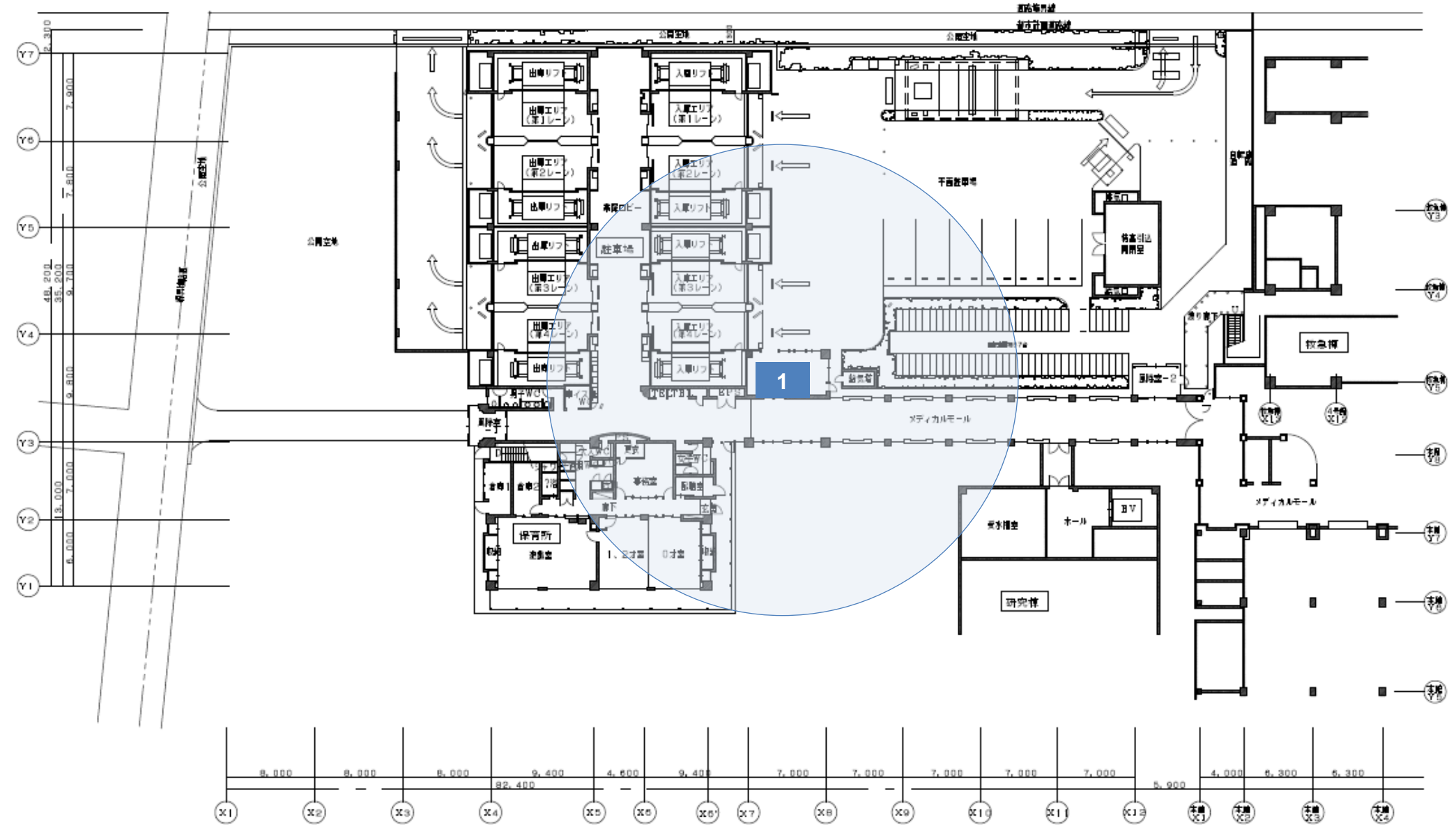
駐車場棟 1階平面図
