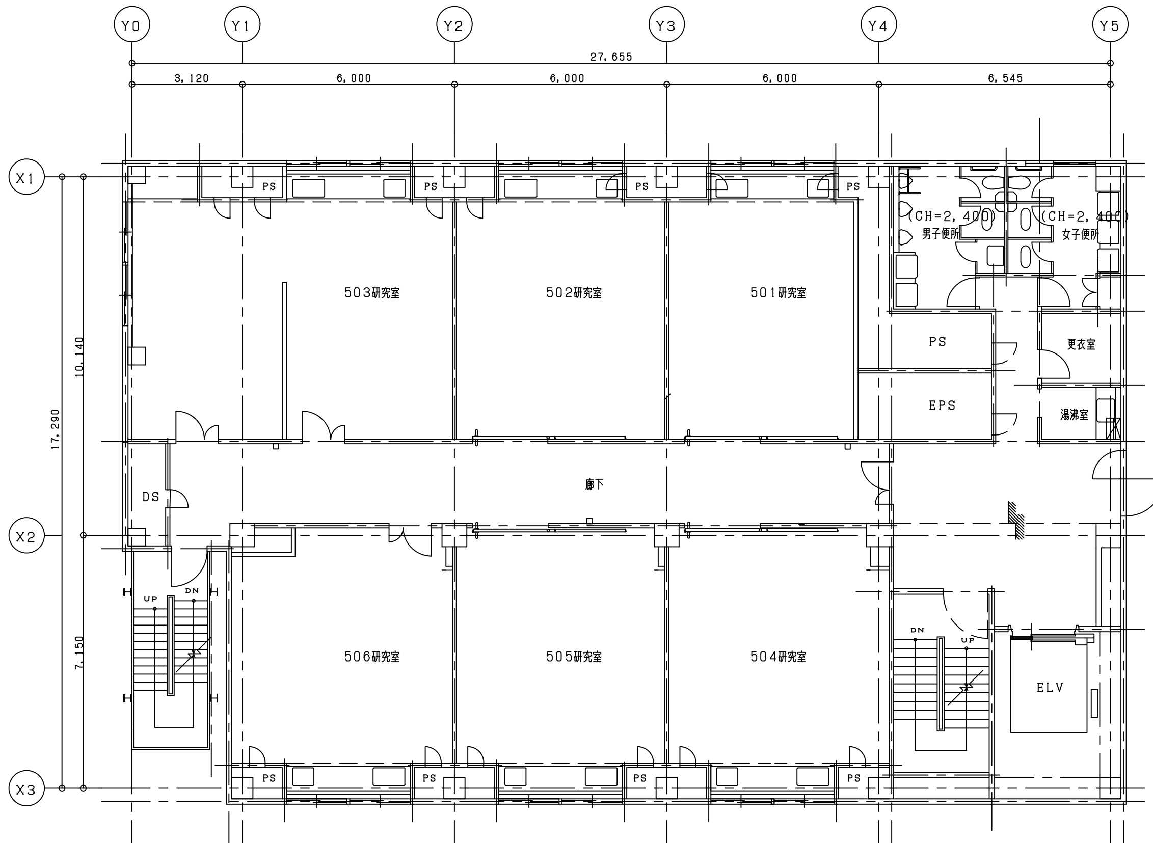
横浜市立大学附属市民総合医療センター研究棟 5階平面図 R1.11 施設担当 1/100 (A3)
