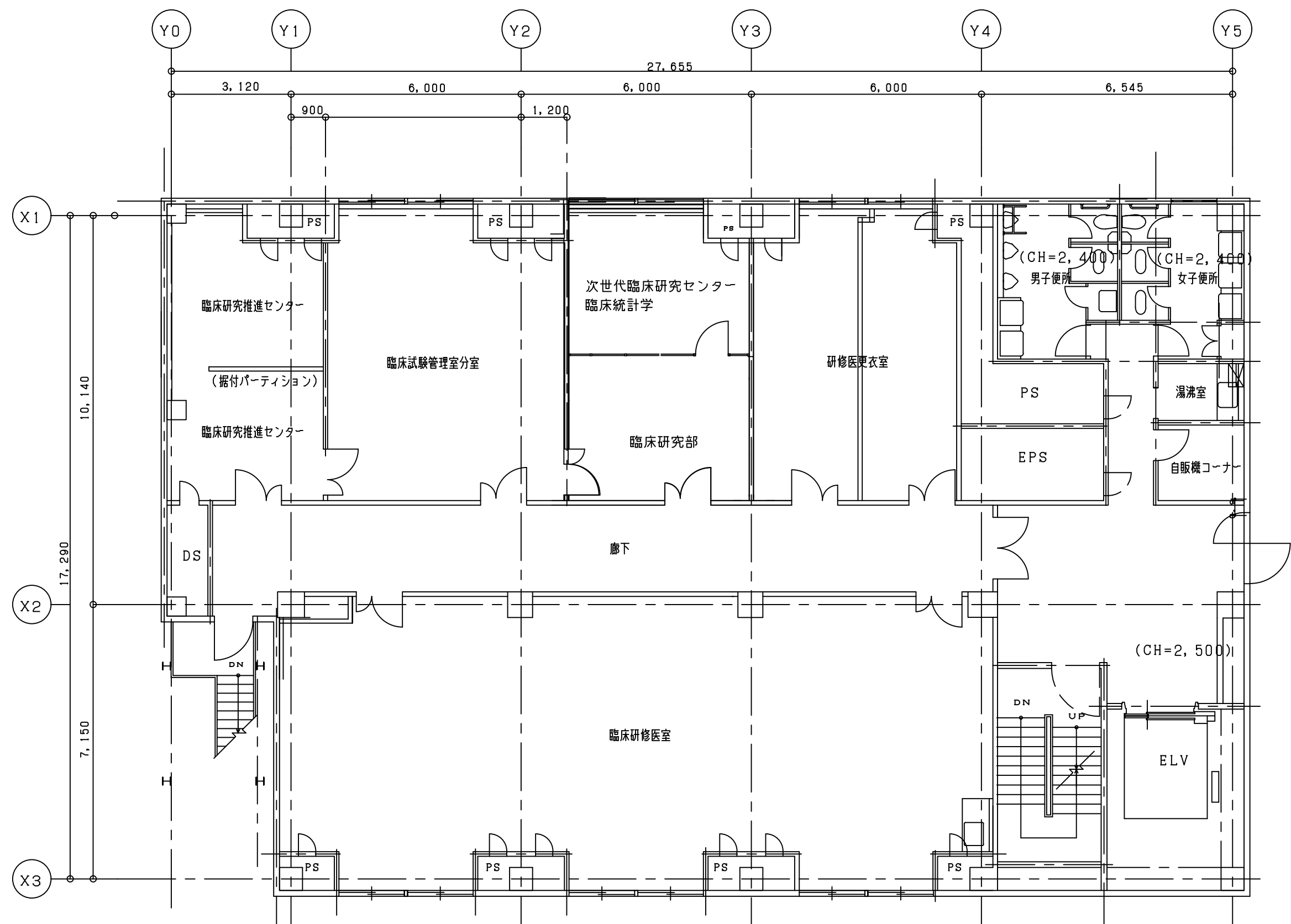
横浜市立大学附属市民総合医療センター研究棟 7階平面図 1/100 (A3) R4.5 施設担当
