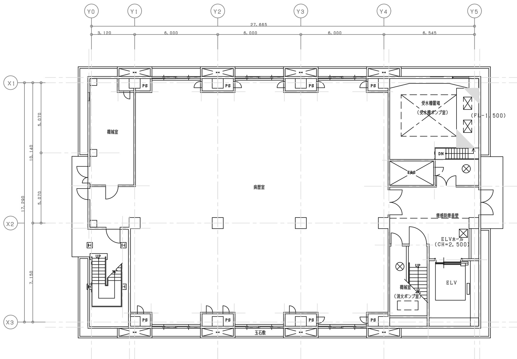
横浜市立大学附属市民総合医療センター研究棟 1階平面図 1/100 (A3)
