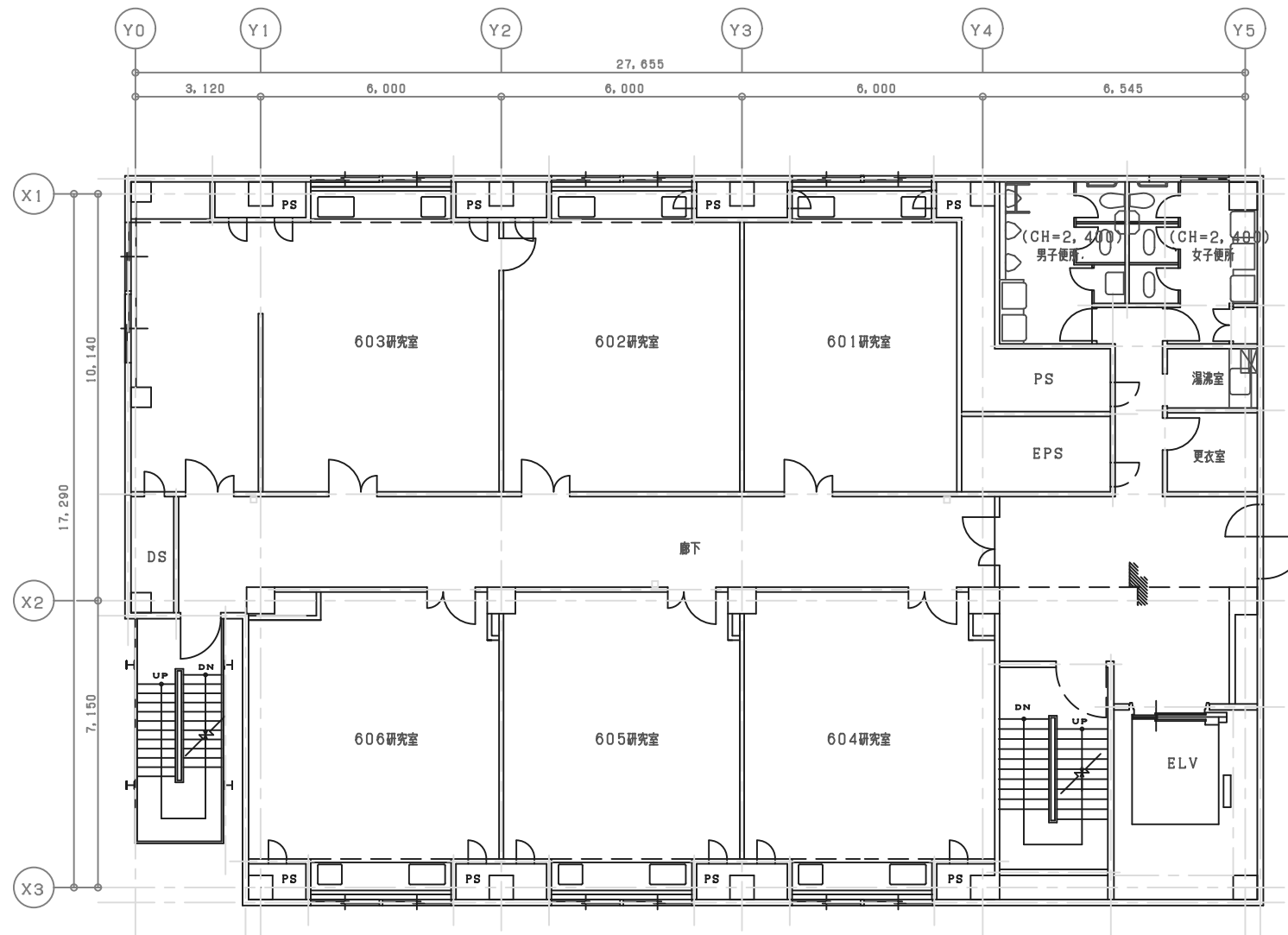
横浜市立大学附属市民総合医療センター研究棟 6階平面図 1/100 (A3) R1.11 施設担当
