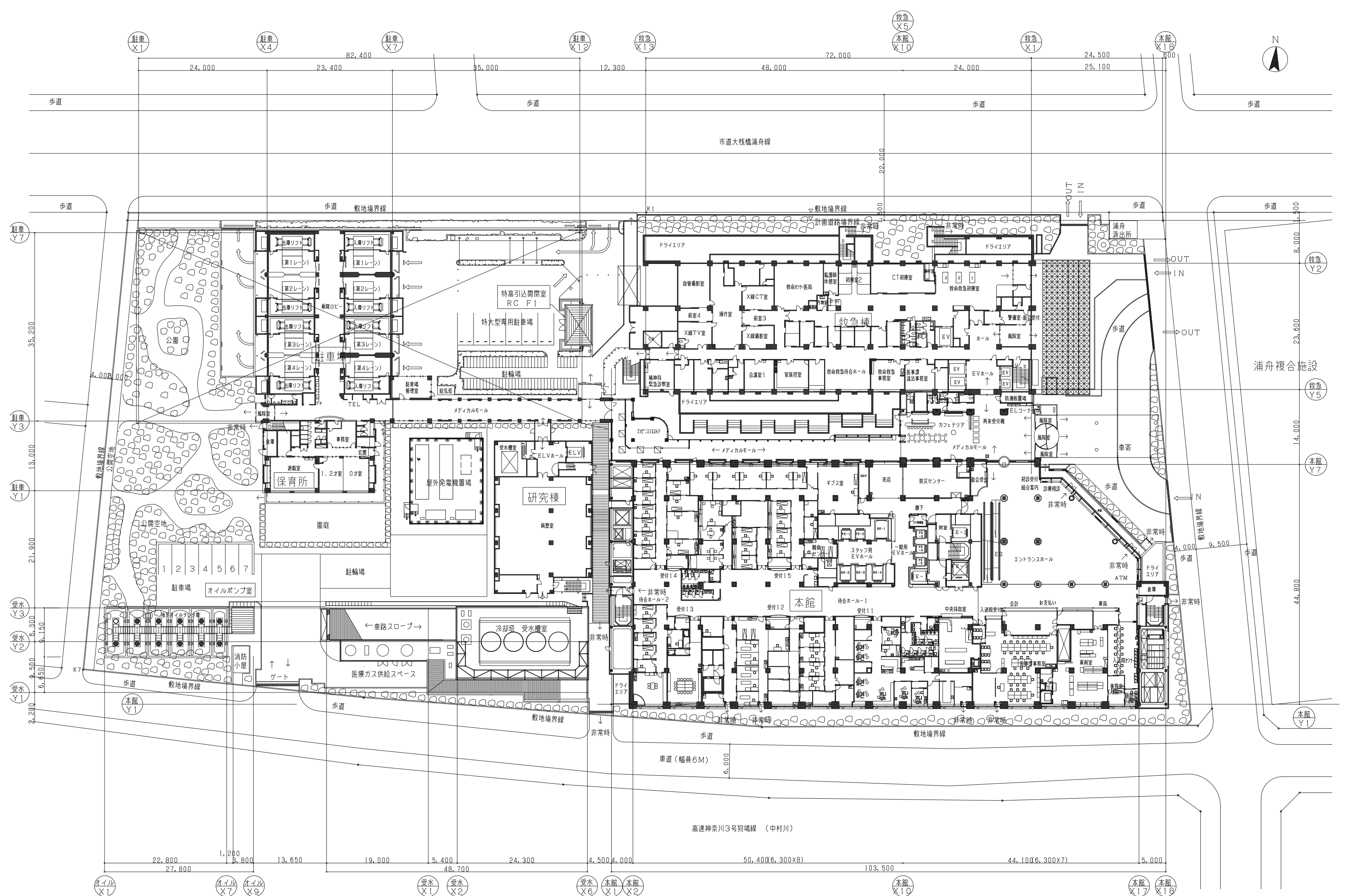
全体配置図
