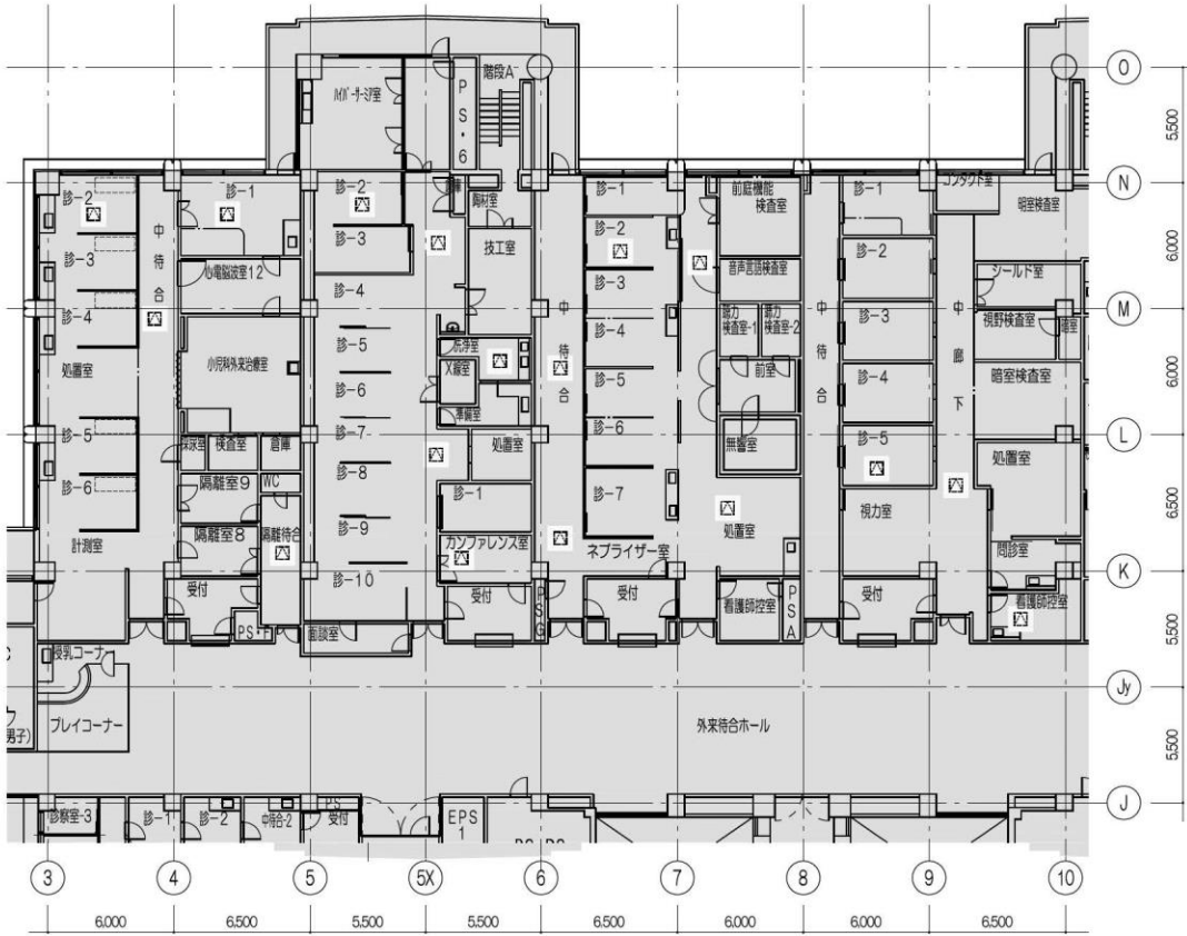
ステップ1：3階撤去・新設工事（13ヶ月の工期の中で天井点検口を設置する）
