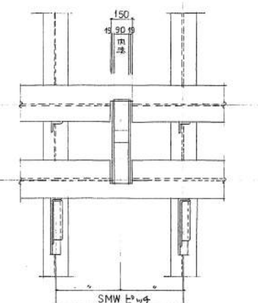
緊張端納り図 ( \theta = 30^\circ ) S-1/20
