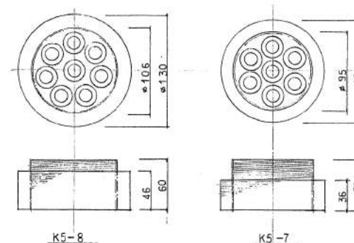
KTBアンカーヘッド S=1/3
