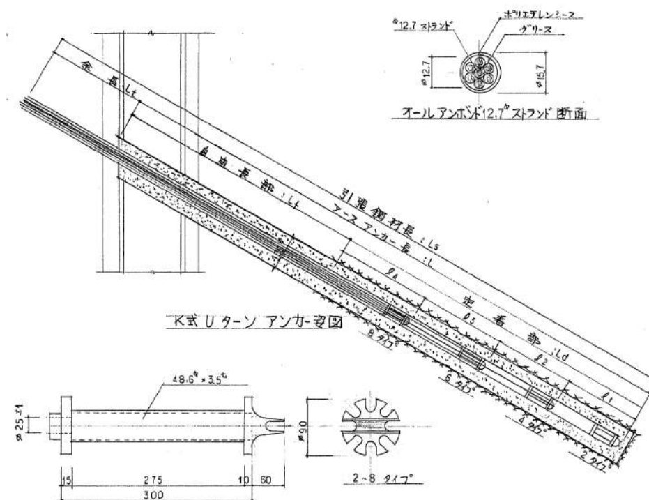
耐荷版詳細図 = 1/40
