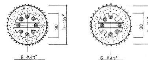
アンカー体 定着部 s=1/3
