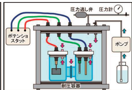
高温高压電気化学装置の開発
