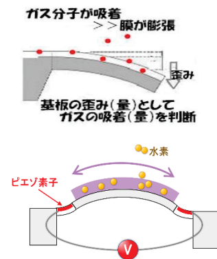
図1 応力検出模式図:カンチレバーの歪として検出するもの(上) MSSのピエゾ素子が検出するもの(下) 吸着分子や高分子に、水素が水素吸蔵膜へ侵入すると、膜を押し広げる力が働き応力が生じる。
