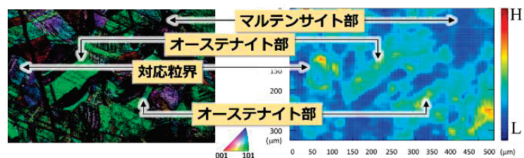
図2 左: ステンレス鋼(SUS304 鋼)表面の構造解析図。右: 同じ位置からの水素像。表面に確認できる結晶粒の形を反映した水素の存在が確認できる。
